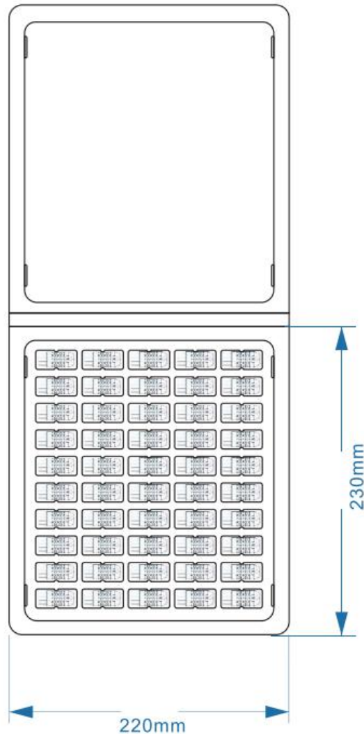
图15. 吸塑盒和传感器定位图
