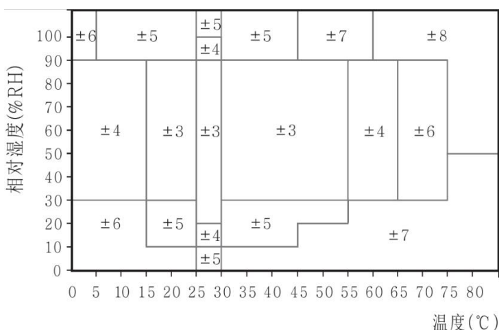
图5. 0~80°C范围内对应的湿度典型误差，单位：(%RH) 请注意：以上误差为以高精度露点仪做参考仪器测试的典型误差（不包括迟滞）。
