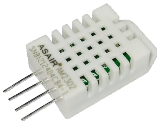
图1. AM2302
