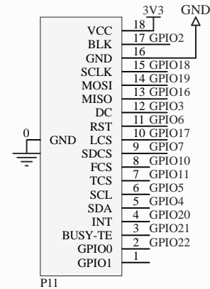
GDI接口
