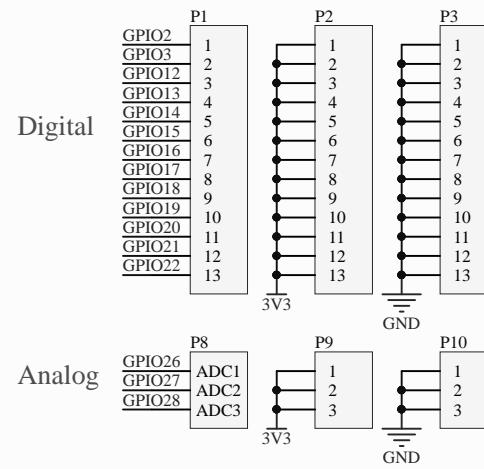
IO扩展口
