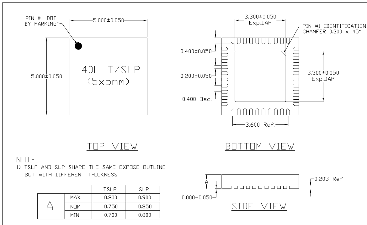
图 6-1. QFN40 (5x5 mm) 封装
