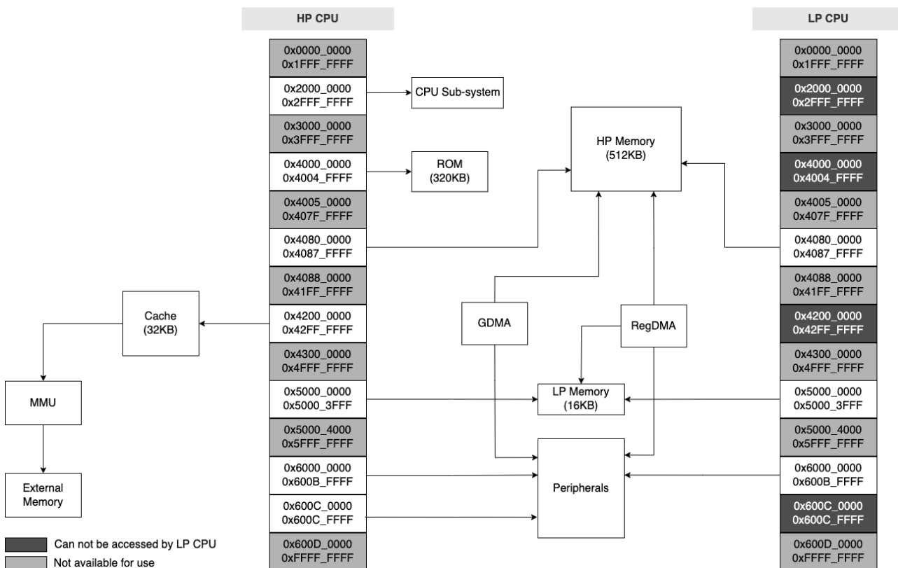
图 3-1. 地址映射结构
