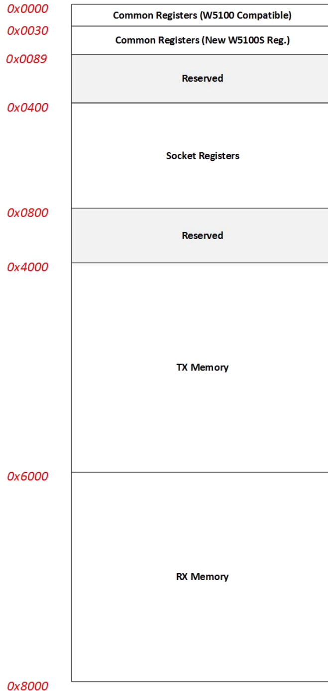
图 3 内存映射表
