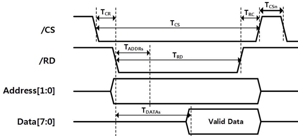
图 26 总线读取时序
