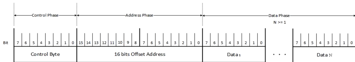
图 17 SPI 帧
