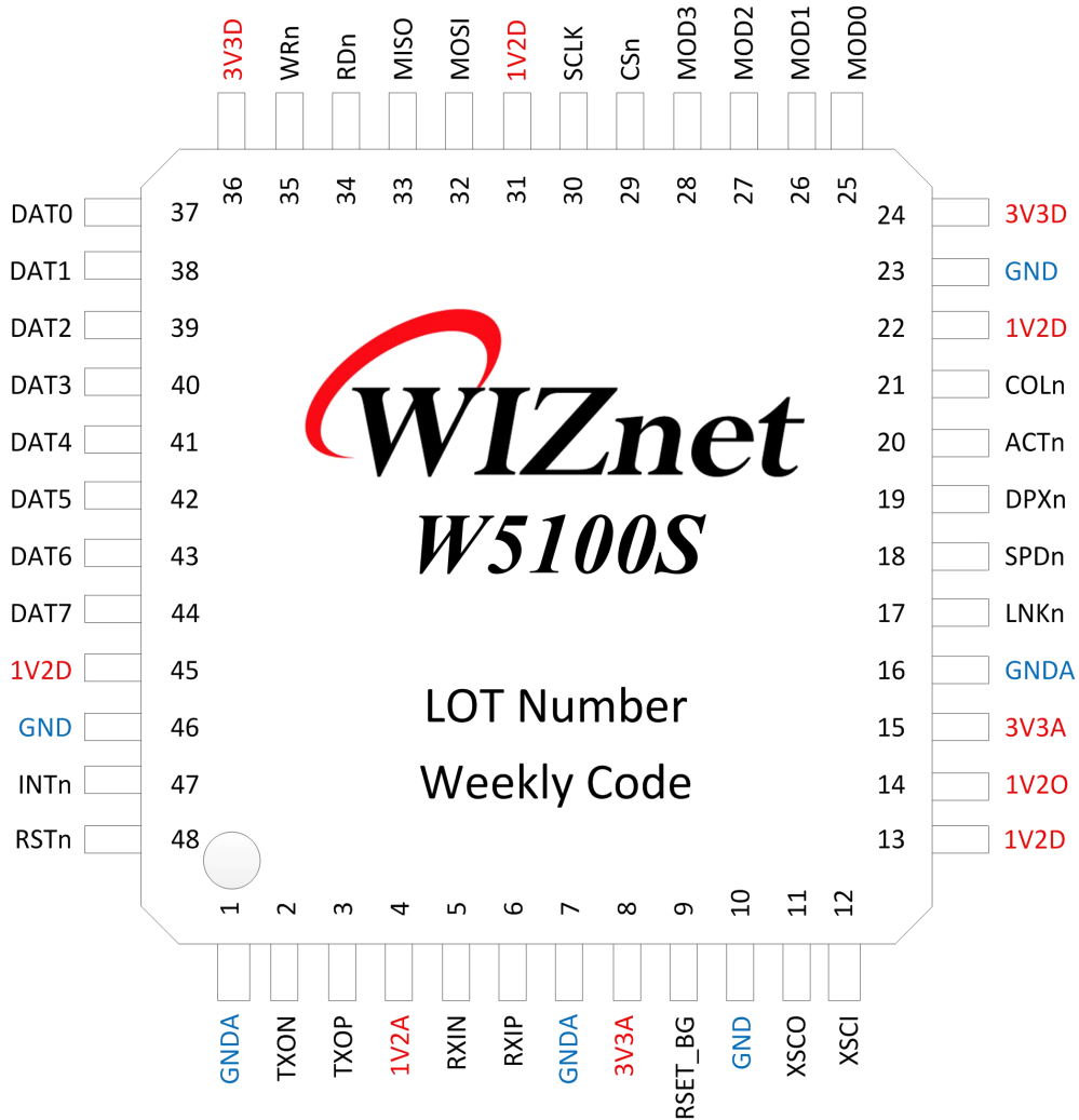
图 2 W5100S 管脚图
