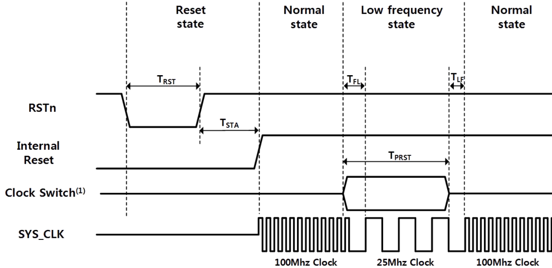
图 25 复位时序
