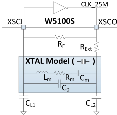
图 23 无源晶振电路模型图
