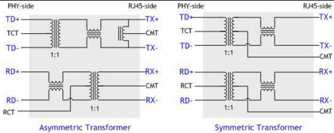
图 30 变压器类型
