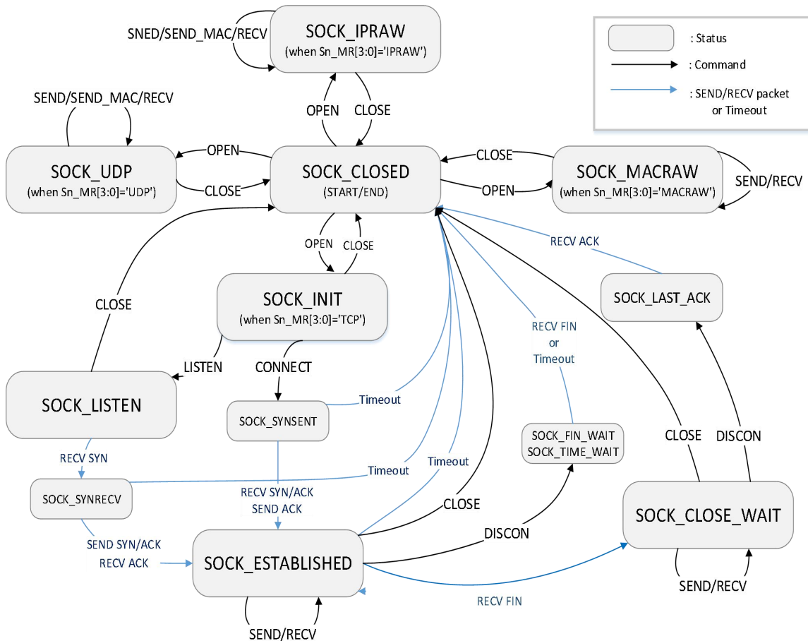
图 4 SOCKET 状态图
