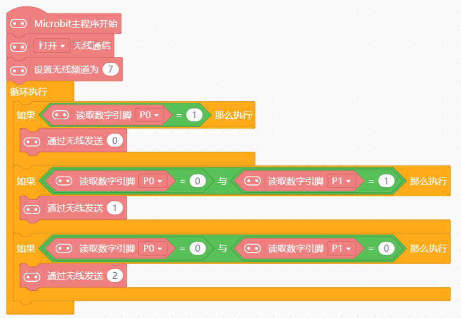
图 4.3.4 发射端执行程序
