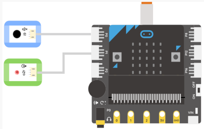
图 3.1.1 接线示意图
