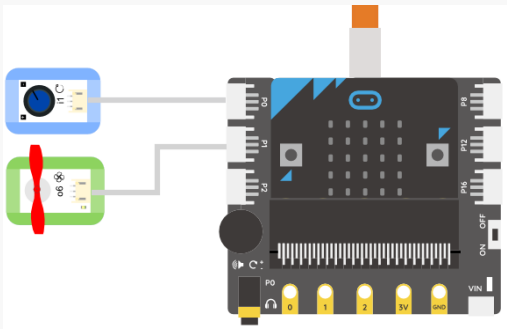
图 2.4.7 连线示意图
