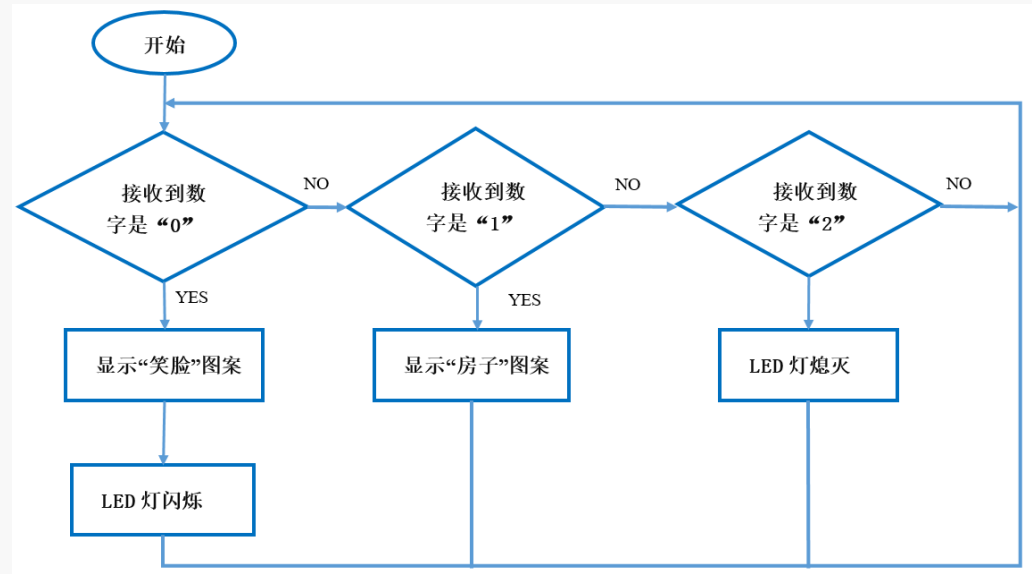
图 4.3.5 接收端逻辑图
