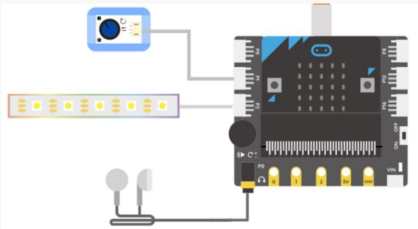
图 4.2.1 连线示意图
