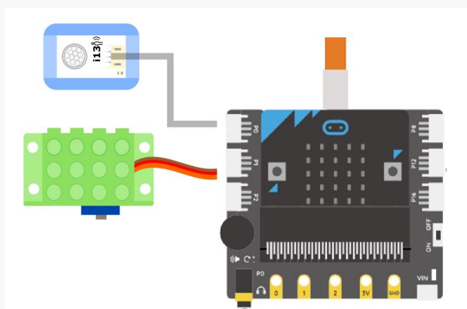
图 3.2.9 连线示意图
