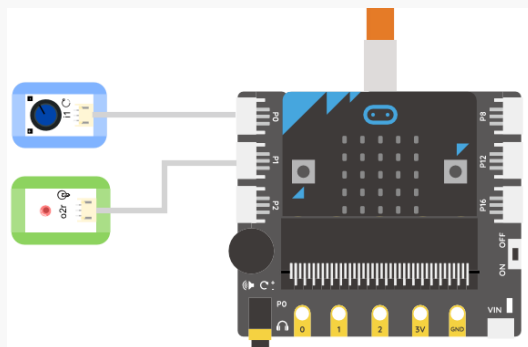
图 2.3.7 连线示意图
