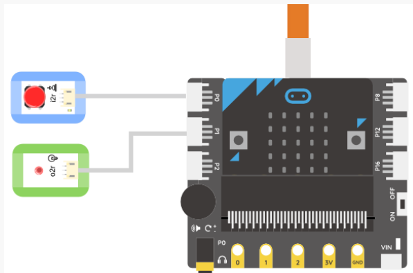
图 2.3.1 接线示意图
