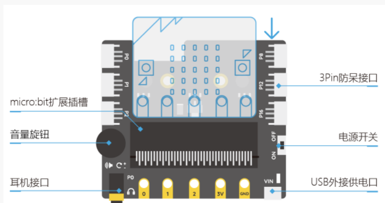
图 1.2.3 micro: bit 扩展板
