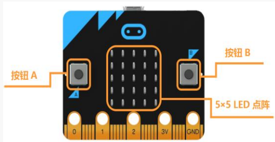
图 1.2.1 micro: bit 正面
