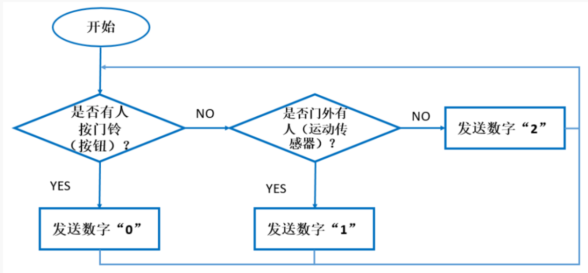
图 4.3.3 发射端逻辑图
