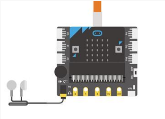
图 3.3.1 接线示意图
