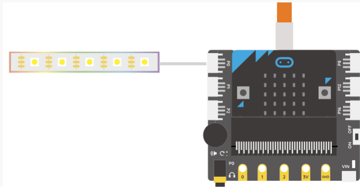
图 4.4.1 连线示意图
