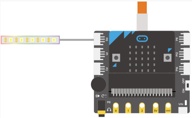
图 3.4.1 接线示意图
