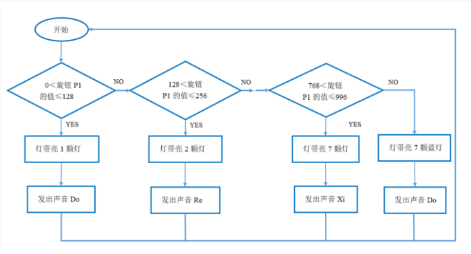
图 4.2.2 逻辑图
