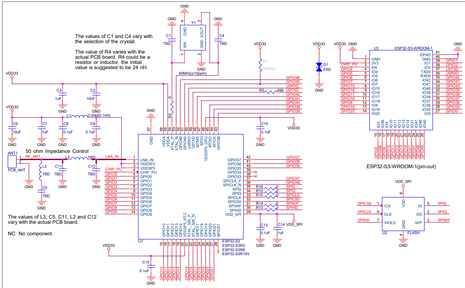
图 5: ESP32-S3-WROOM-1 原理图
